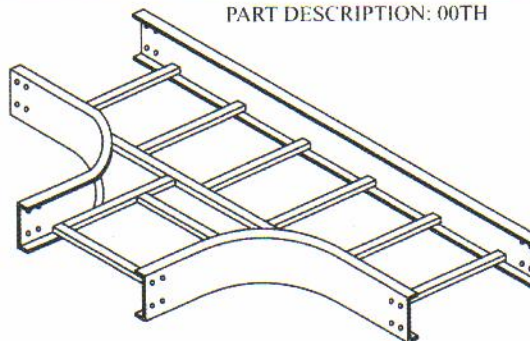
HORIZONTAL Tee
